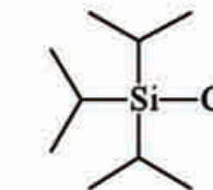
Triisopropylchlorosilane
