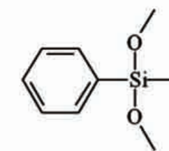
Dimethoxymethylphenylsilane
